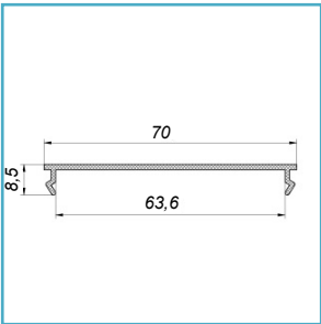
Розсіювач РС 70 матовий, з полікарбонату. L = 2000 мм.
