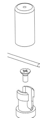
Комплект КТ4 Зажим для кріплення конструкції до троса.
