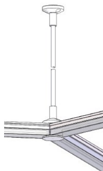
Комплект КТ13 Для з'єднання профілів у підвісній конструкції. Використовується разом з комплектами КТ21 та КТ22.
