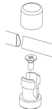
Комплект КТ1 Зажим для кріплення конструкції до труби.
