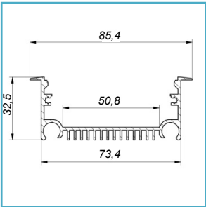
Профіль алюмінієвий анодований, колір — срібло. L = 2000 мм. P = 498 мм.
